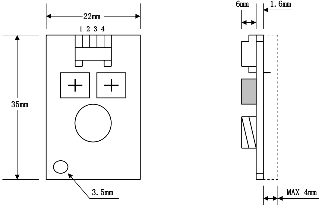
图 1. 外形图 (SC0083 型) .
