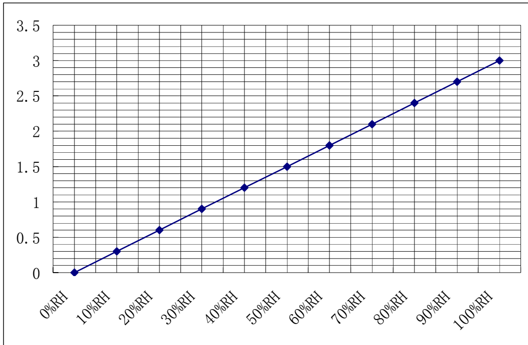
图 4. 标准特性图
